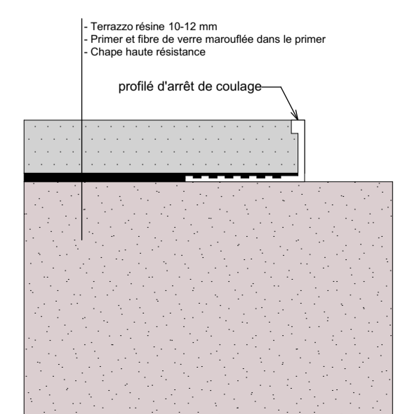
ARRÊT DE COULAGE
