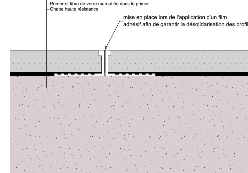
JOINT DE FRACTIONNEMENT
